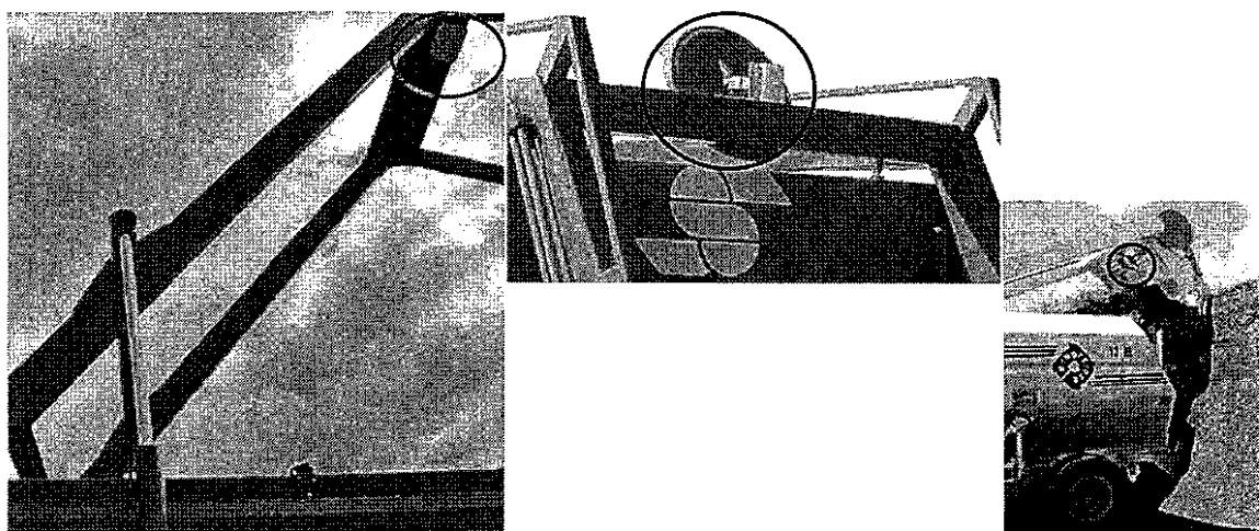
Figura 15. Esempi applicativi di specchi (evidenziati in figura) installati sulla struttura portante dei bracci dell'organo di taglio (fresa).
