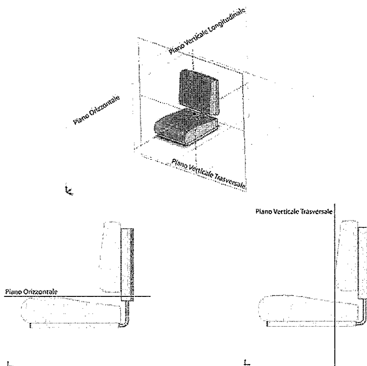
Figura 3. Individuazione del punto S del sedile
