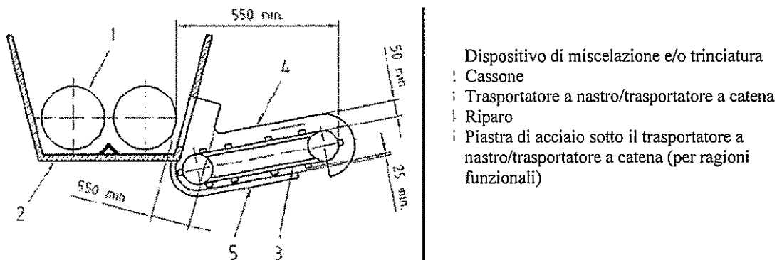
Figura 7. Protezione contro l'accesso diretto all'apertura di scarico quando è posizionata lateralmente (caso di un trasportatore con catena di acciaio). Dimensioni in mm.
