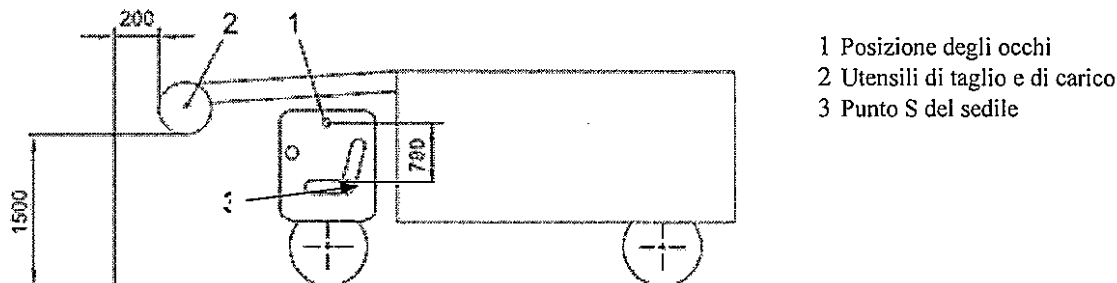
Figura 1. Area di lavoro per la verifica della visibilità diretta per le macchine semoventi. Dimensioni in mm.
