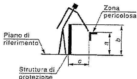
Figura 11. Accessibilità al di sopra di strutture di protezione.
