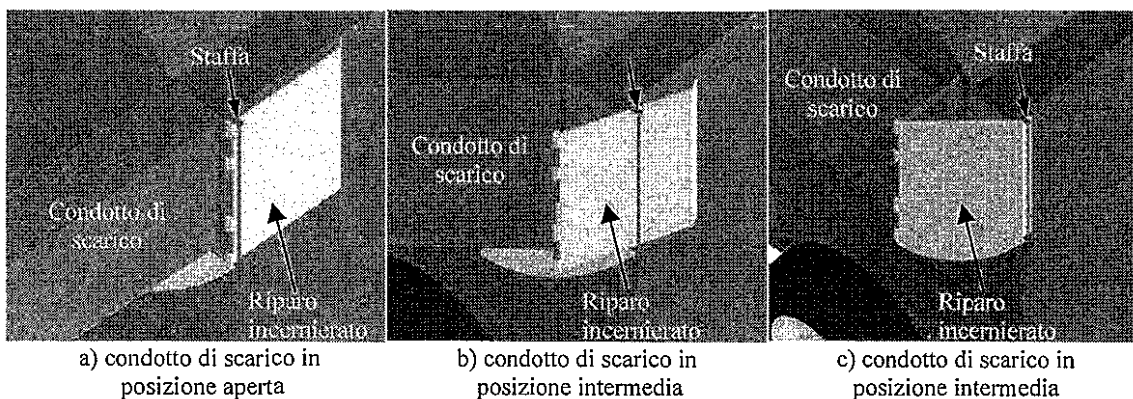
Figura 22. Riparo incernierato collegato al condotto di scarico
