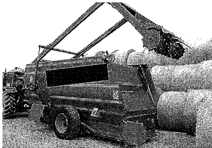
Figura 20. Organi di taglio e di carico in posizione sollevata: parete mobile in posizione abbassata ed organi di miscelazione e/o trinciatura in movimento protetti.
