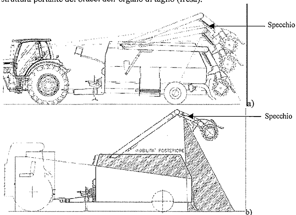
Figura 14. Visibilità posteriore ottenuta con l'installazione di uno specchio sul braccio fresa.
