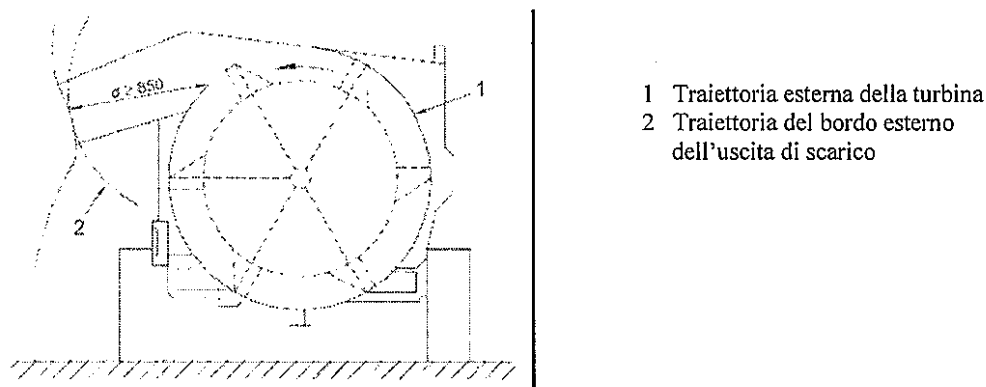
Figura 10. Protezione contro il pericolo di pizzicamento con le turbine. Dimensioni in mm.
