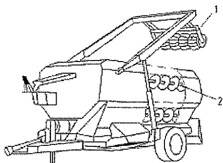
c) Carro desilatore trainato orizzontale
