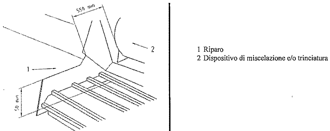
Figura 6. Protezione del nastro trasportatore mediante riparo pieno. Dimensioni in mm.
