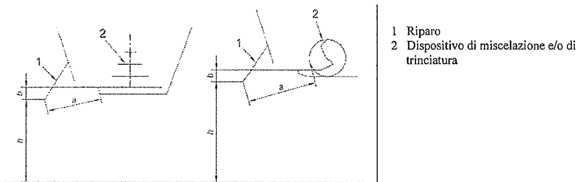
Figura 9. Protezione contro il pericolo di pizzicamento con il dispositivo di miscelazione e/o trinciatura in caso di scarico libero.
