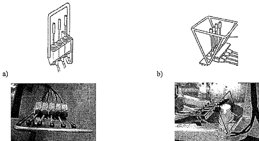
Figura 16. Esempi di protezione delle leve contro l'azionamento accidentale
