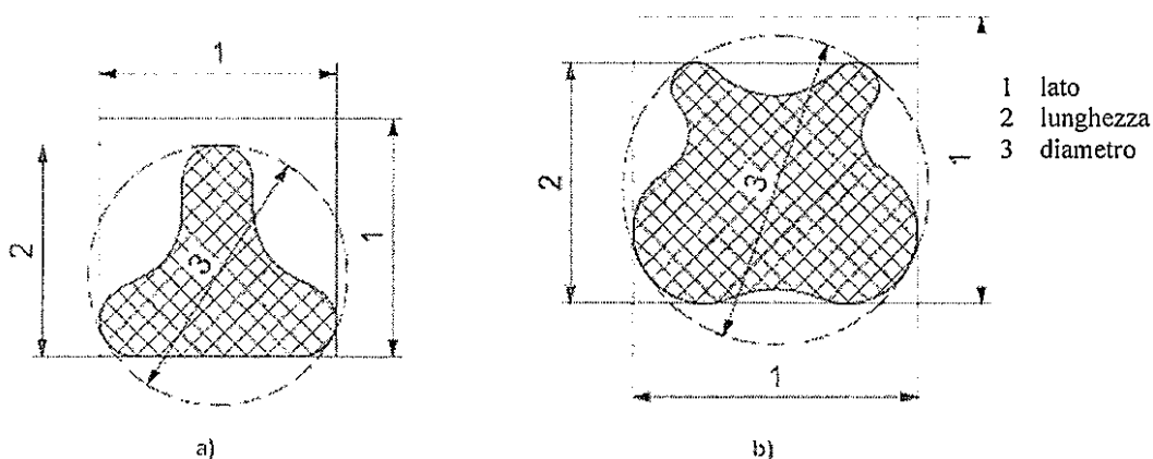
Figura 12. Esempi di aperture di forma irregolare.
