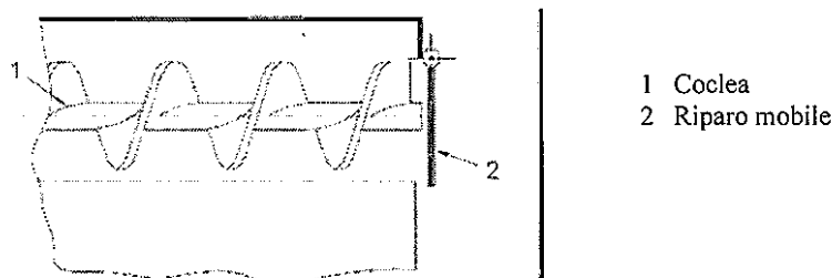
Figura 8. Riparo mobile a chiusura automatica per la protezione della coclea.
